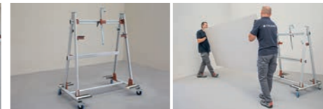
CARRELLO DI MOVIMENTAZIONE predisposto per eseguire la stesura della colla sul retro lastra. HANDLING TROLLEYS designed to allow application of adhesive to the back of the slab.
