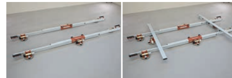
BARRE / TELAIO DI MOVIMENTAZIONE con ventose per formati fino a 160x320 cm. SUCTION CUP HANDLING BARS / FRAME for sizes up to 160x320 cm.
